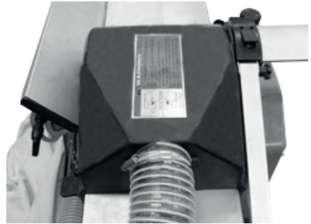
Fig. 12 – Instalación de la caja colectora de polvo sobre las cuchillas
