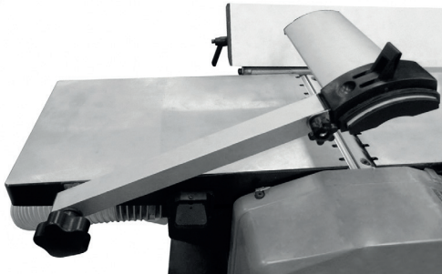
Fig. 11 – Brazo de la guarda de protección
