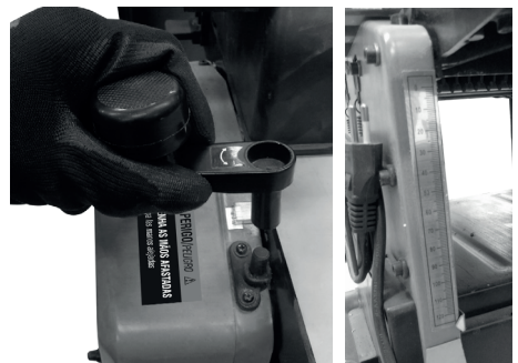
Fig. 13 – Ajuste de la mesa en el modo afinado
