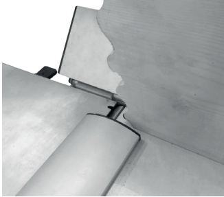
Fig. 7 – Ajuste da guarda de proteção
