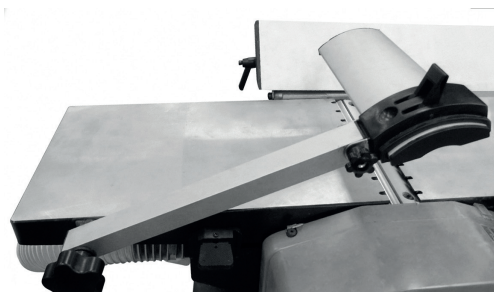
Fig. 11 – Braço da guarda de proteção
