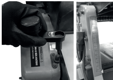
Fig. 13 – Ajuste da mesa no modo desengrossadeira
