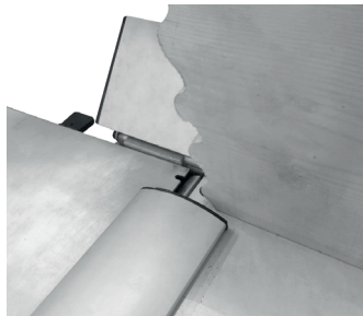
Fig. 7 – Ajuste la guarda de protección
